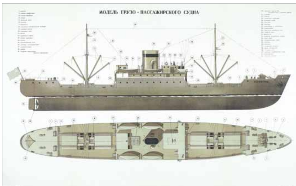
Лот № 205. Плакат «Модель грузо-пассажирского судна». М.: 5-я литография, 1951. 57 × 92 см. В коллекционном состоянии.
